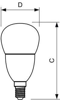
Candle WG EMEA 60W E14 P50
