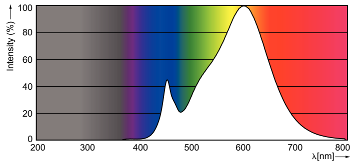
A60 /830 FR
