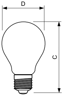
filament 7.5W-60W 806lm NAD 2700K E27ND
