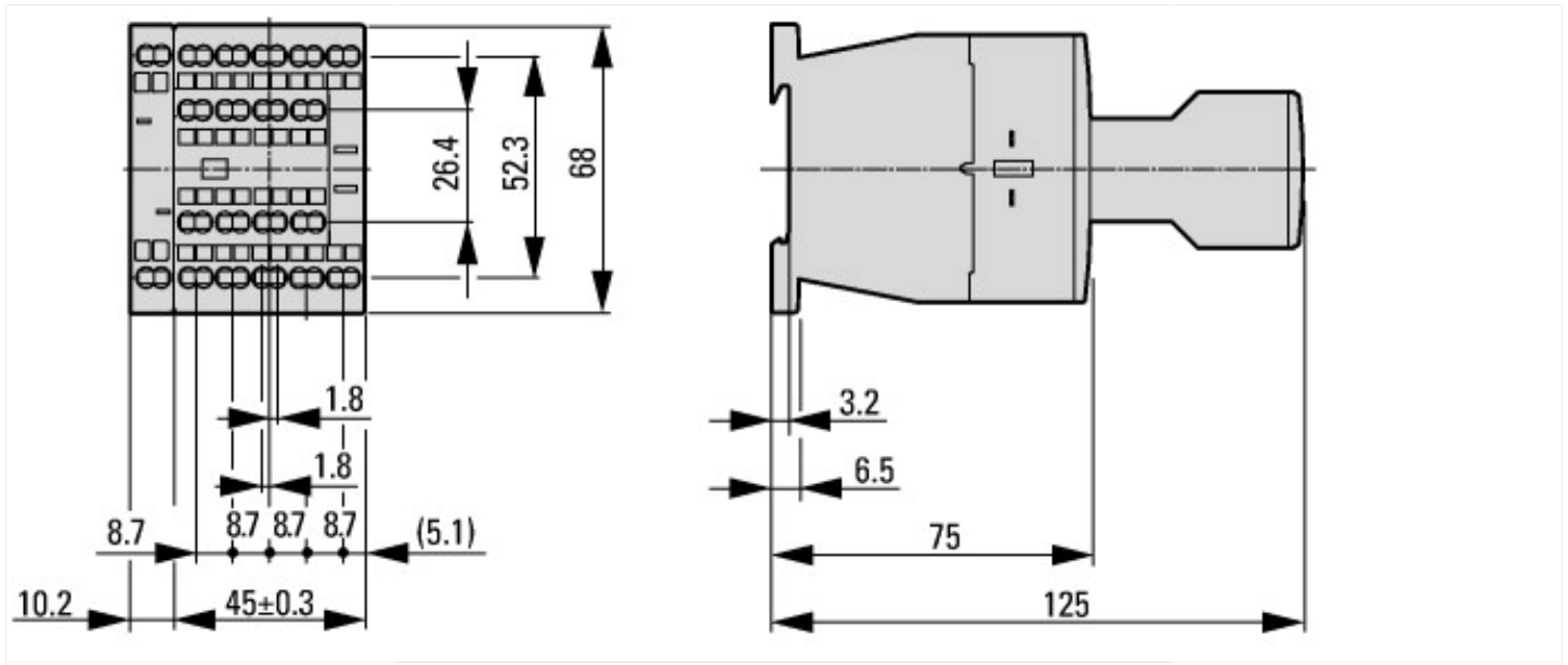
Contacteur with auxiliary contact module
