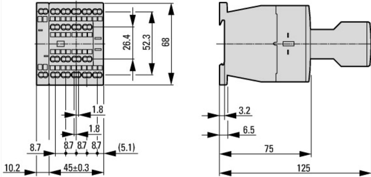
Contacteur with auxiliary contact module
