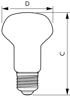
R63 220-240V 5.5-40W 400lm 2700K E27 Dim
